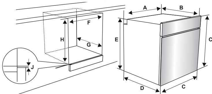
Installering under en benkeplate
