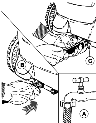
Wasseranschluß.
