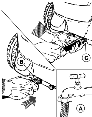
Collegamento idrico.
