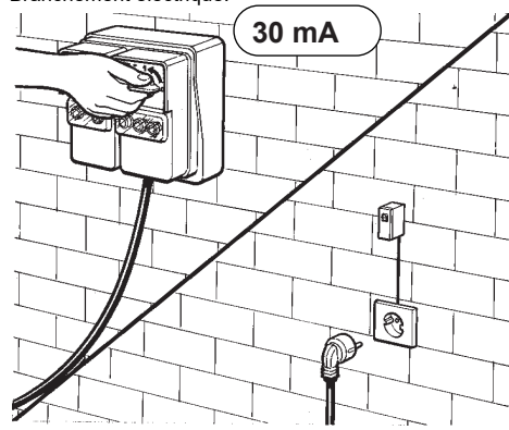
Branchement électrique.
